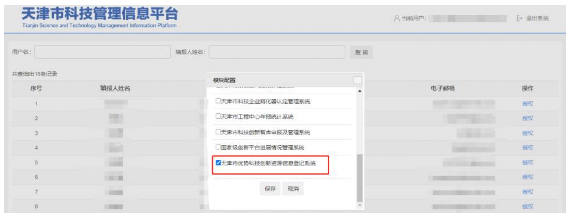
图 2-11 授权配置
