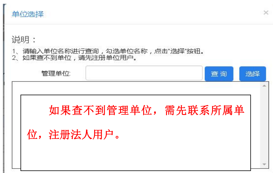
图 2-9 单位选择
