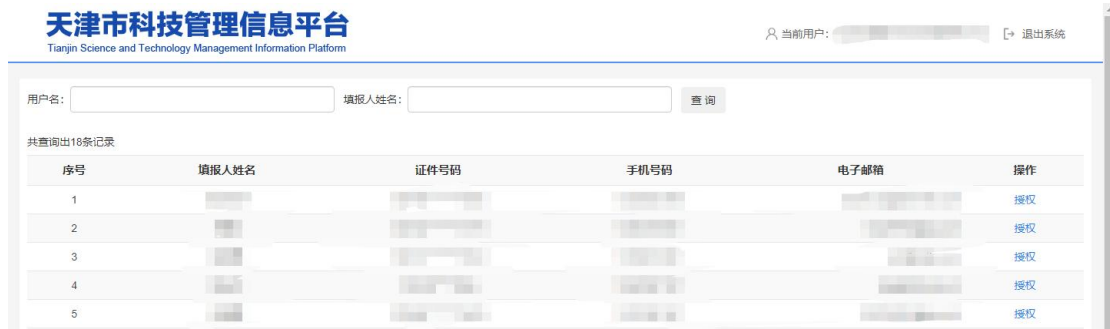
图 2-10 登录页面
